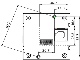
图 2-2-D 小键盘底座安装尺寸
