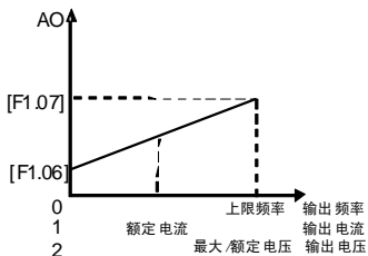
图 6-7 模拟输出端子的模拟输出内容
