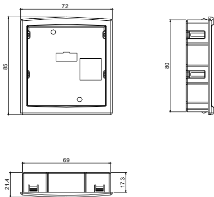
图 2-2-E 小键盘安装底座尺寸
