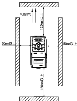
图 2-1-A 安装的间隔距离
