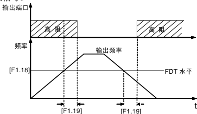
图 6-10 频率水平检测信号 (FDT)
