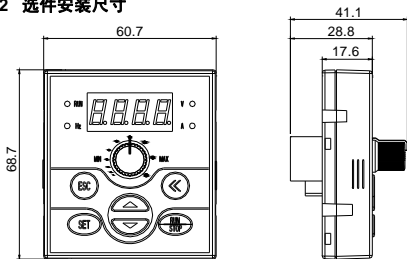
图 2-2-C 小键盘安装尺寸
