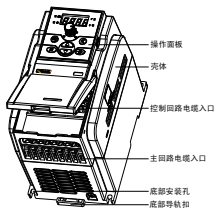
图 1-2 II类变频器外观及部件名称
