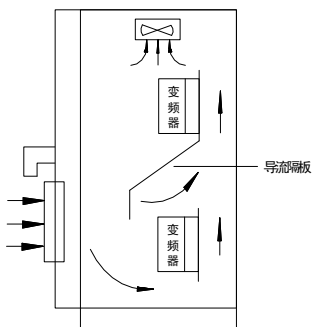
图 2-1-B 多台变频器的安装
