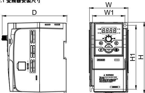
图 2-2-A 变频器安装尺寸 1
