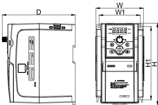
图 2-2-B 变频器安装尺寸 2
