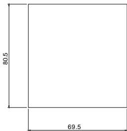
图 2-2-F 小键盘安装底座开孔尺寸
