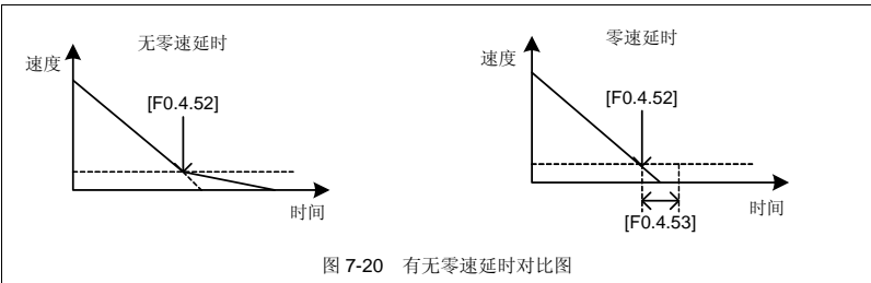
图 7-20 有无零速延时对比图
