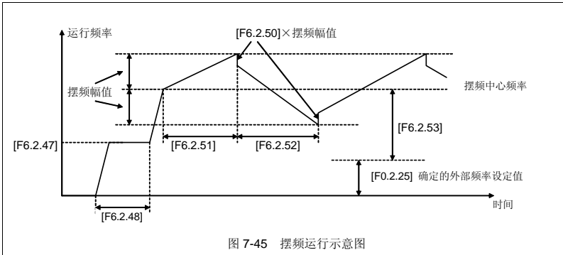
图 7-45 摆频运行示意图
