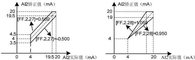
图 7-61-A A12 零偏矫正曲线
