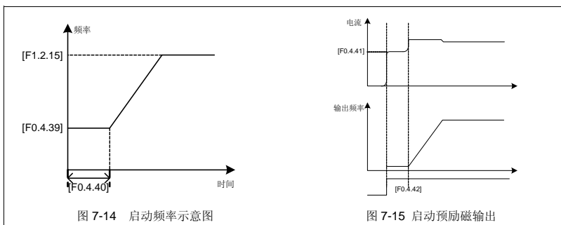
图 7-14 启动频率示意图
