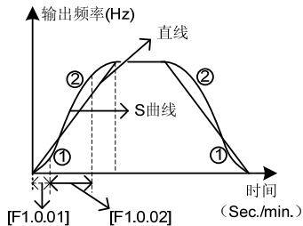
图7-21 加减速曲线
