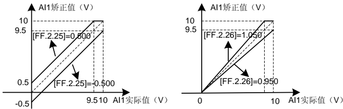
图 7-60-A A11 零偏矫正曲线
