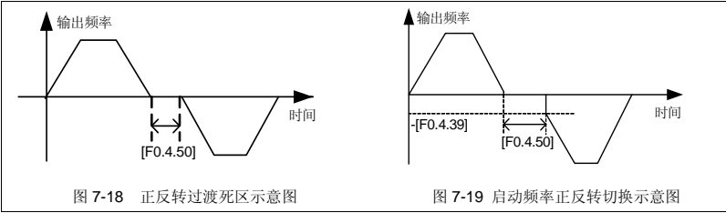
图 7-18 正反转过渡死区示意图
