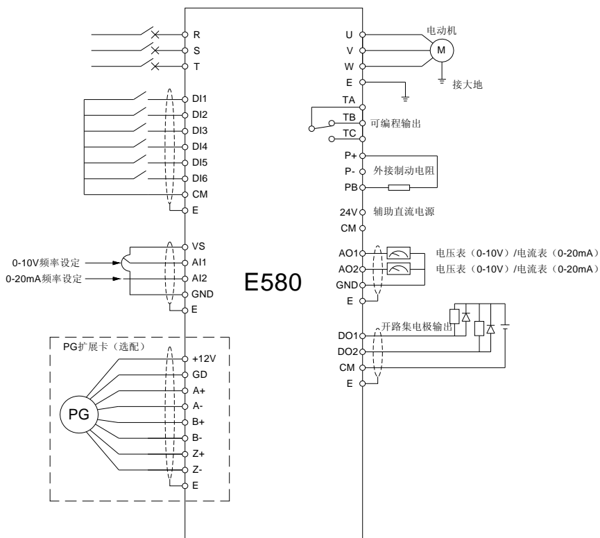
图 4-2 E580 系列变频器基本接线图
