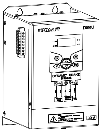
图 12-2 外观示意图
