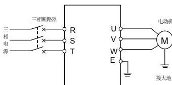
图 5-3 SVC 运行接线
