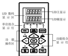
图 5-1-B 双行 LED 标准操作面板
